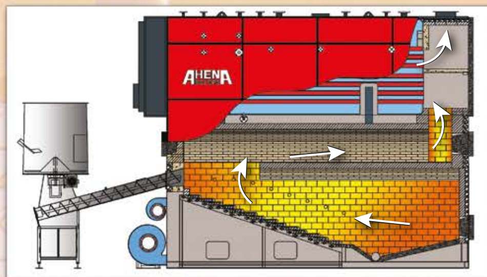
Caldaie a griglia mobile con basamento a secco e caricamento a coclea/spintore Moving grate boilers with dry base and screw/pusher feeding
