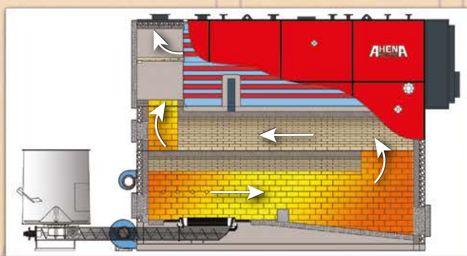
Caldaie con bruciatore meccanico a coclea sottoalimentato in basamento a secco Boilers with mechanical screw burner installed in dry base
