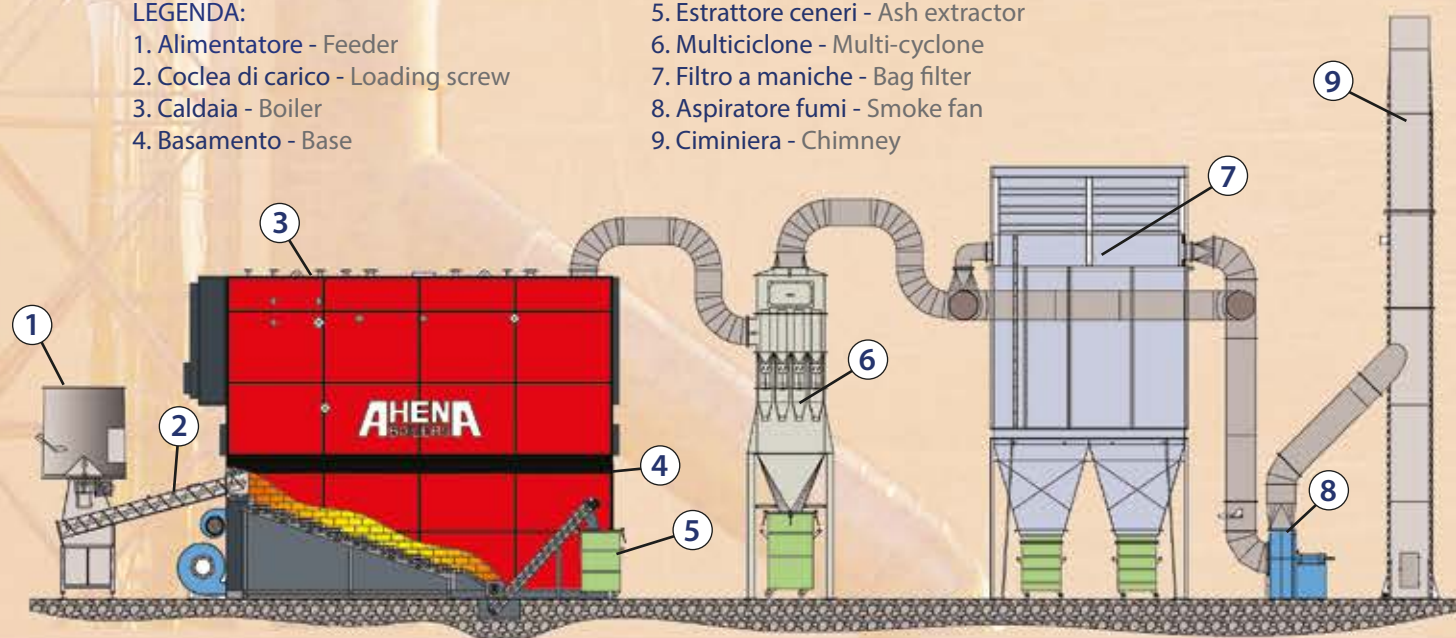
Caldaie con bruciatore meccanico a coclea sottoalimentato in basamento a secco Boilers with mechanical screw burner installed in dry base
